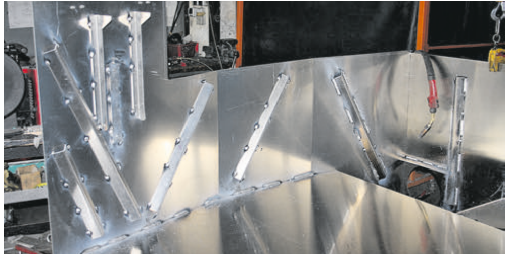
Hier entsteht ein großer Tank, die Verstrebungen an der Innenseite sorgen später für die Stabilität.
